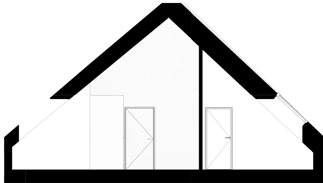
Snit gennem bolig, snit A-A
