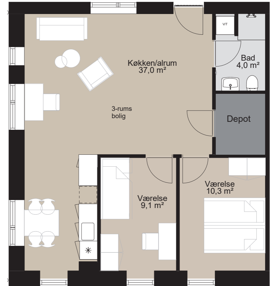
Plantegning
