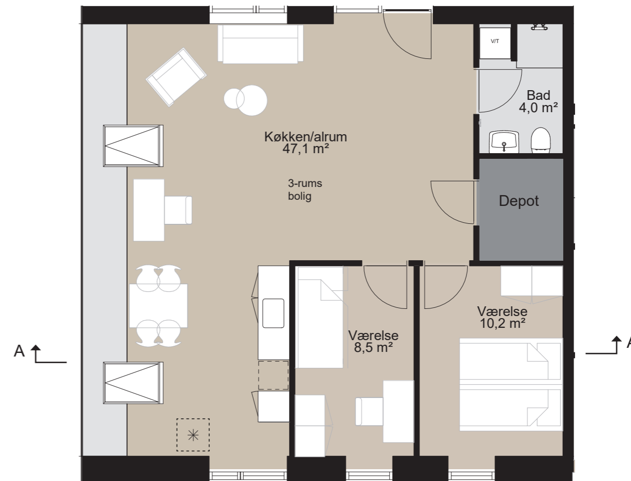
Plantegning
